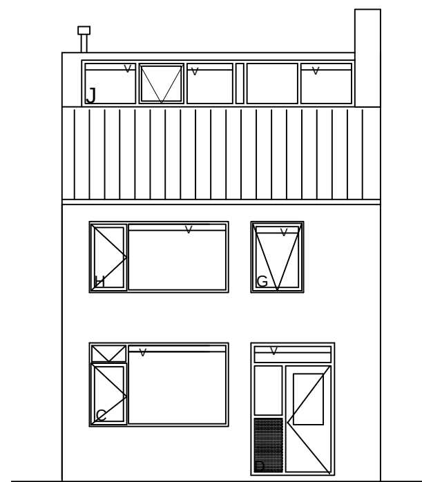
ACHTERGEVEL
