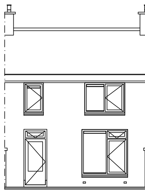
Achtergevel
