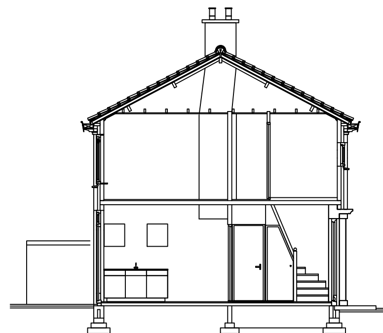
Doorsnede
