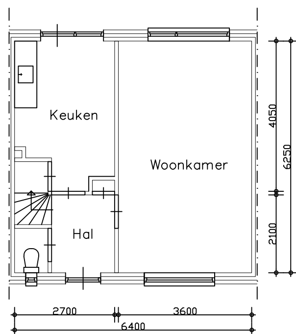
Begane grond
