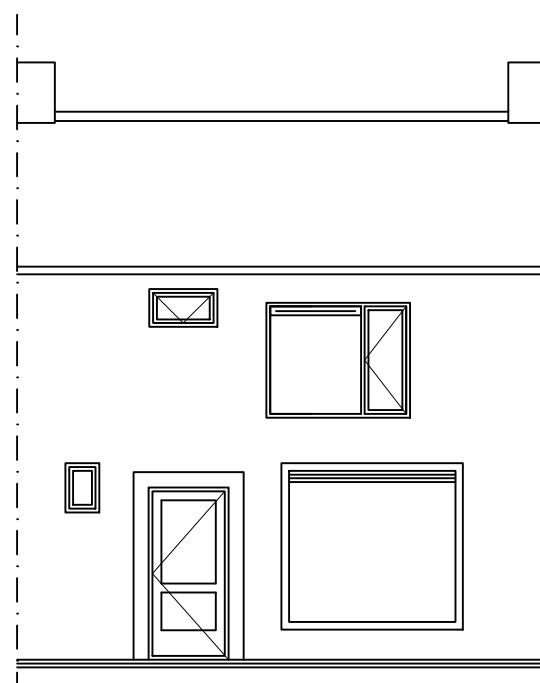
Voorgevel
