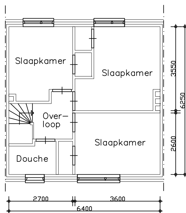
Verdieping
