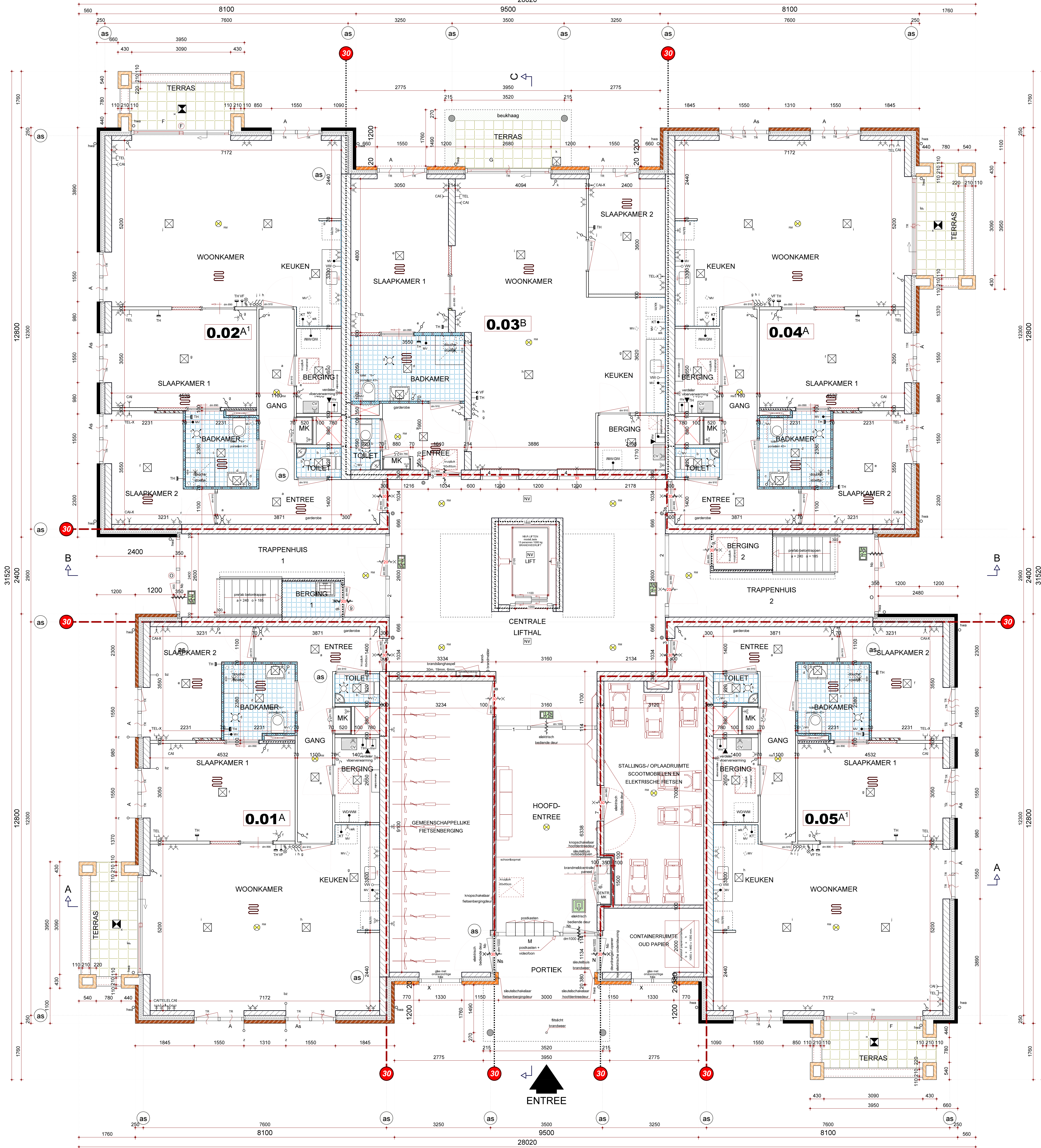
BEGANE GROND
