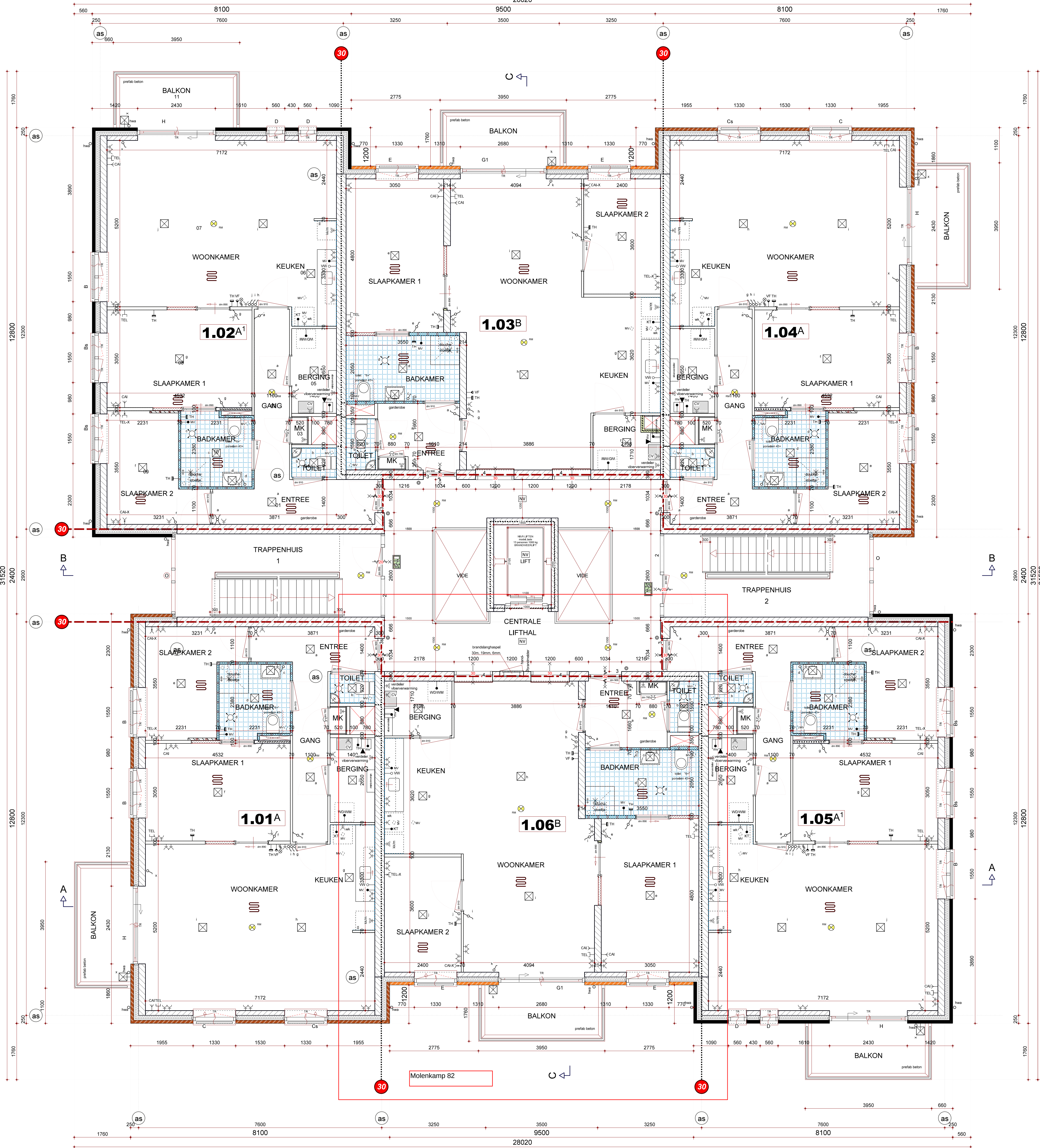
1e VERDIEPING
