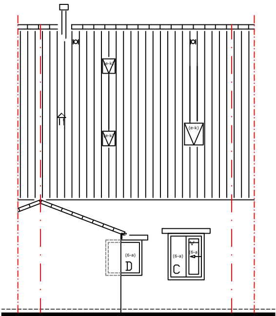
ACHTERGEVEL
