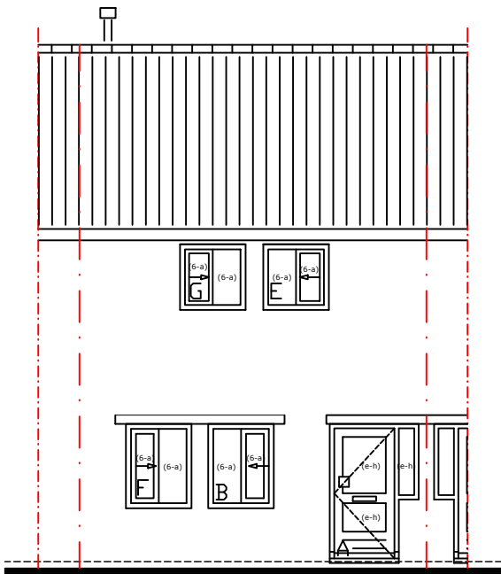
VOORGEVEL
