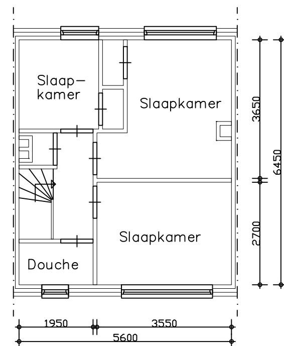
Verdieping
