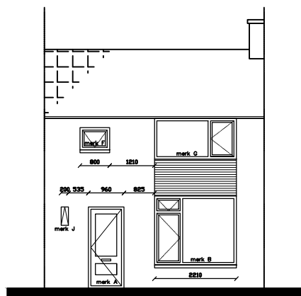
Voorgevels
