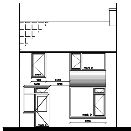
Achtergevels
