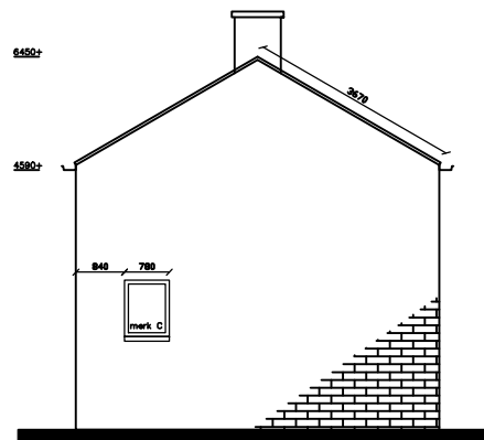
Kopgevel
