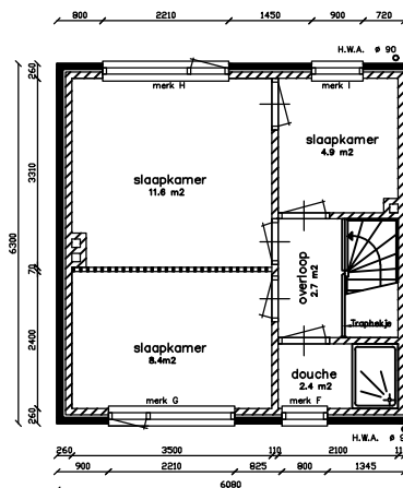
Verdieping
