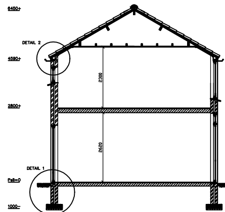
DOORSNEDE schaal 1:50
