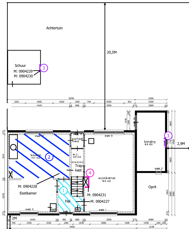
Begane Grond
