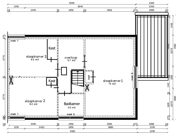
Eerste verdieping
