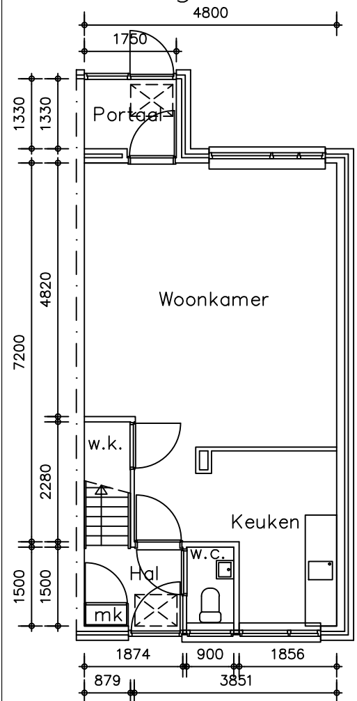
Beganegrond
