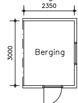
Plattegrond
