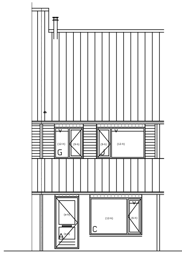
VOORGEVEL
