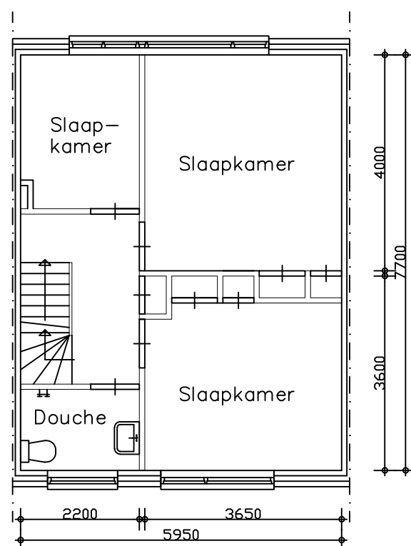
Verdieping
