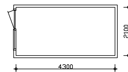
Plattegrond Berging
