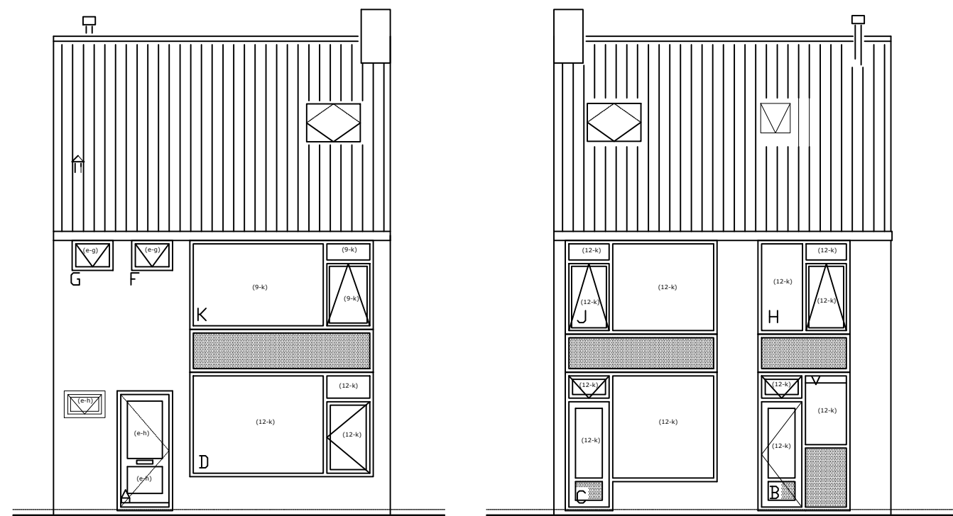
VOORGEVEL
