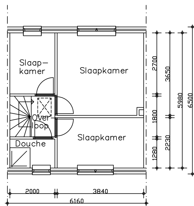
Verdieping
