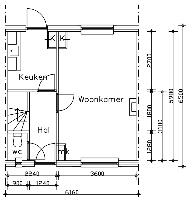
Begane grond
