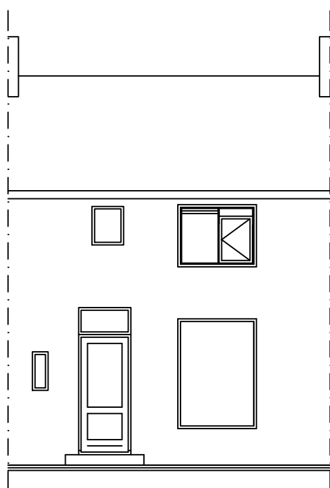
Voorgevel
