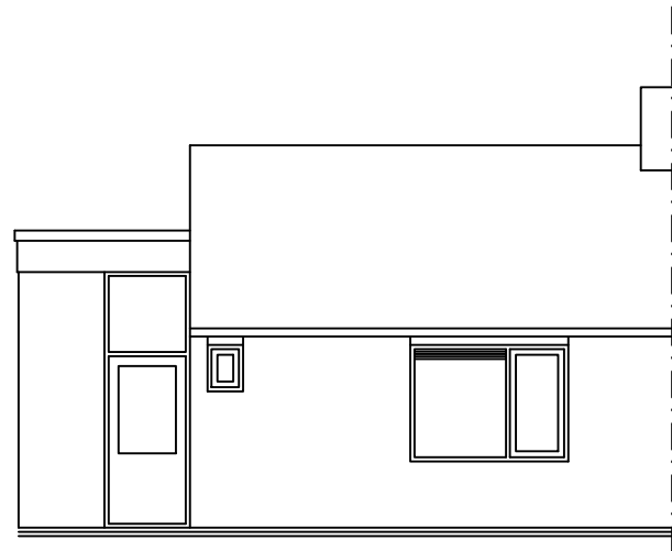
Zijgevel
