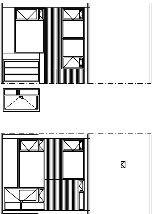
Voorgevel
