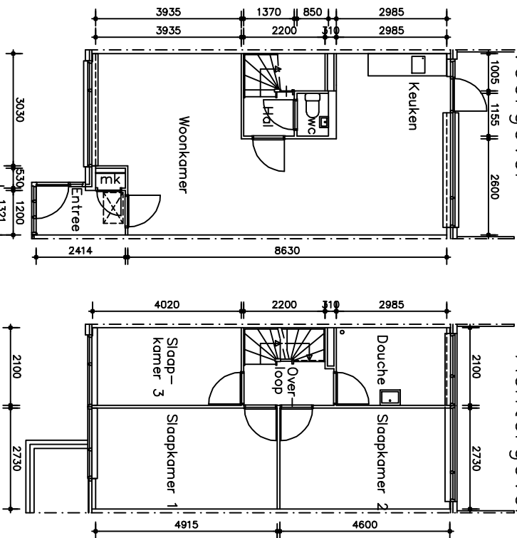
Beganegrond
