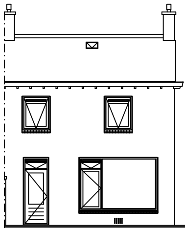
Achtergevel
