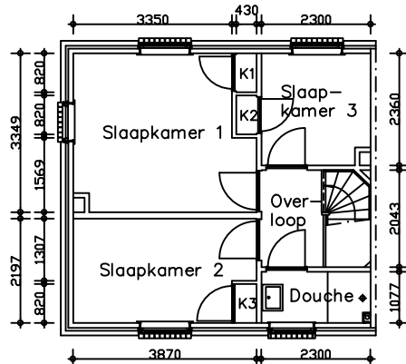
Verdieping
