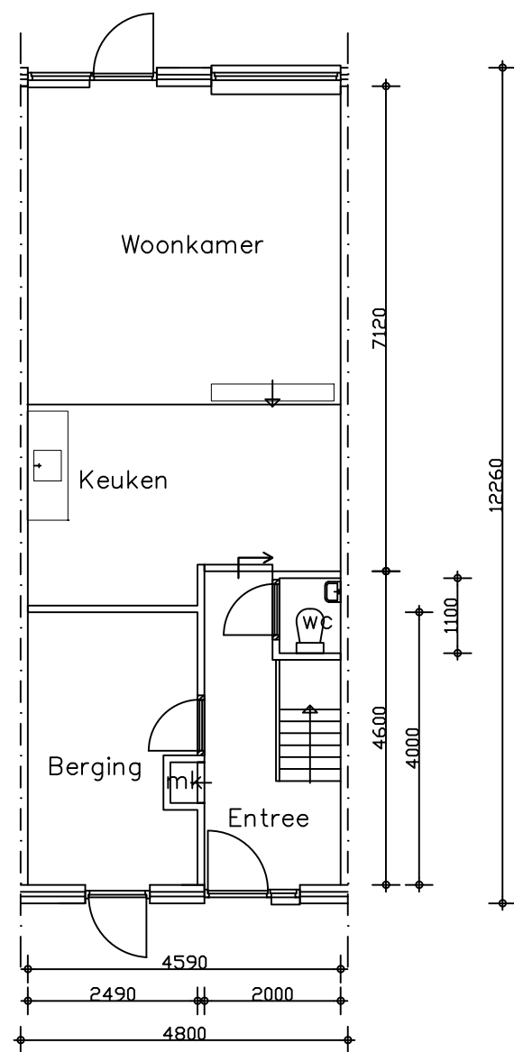
Beganegrond
