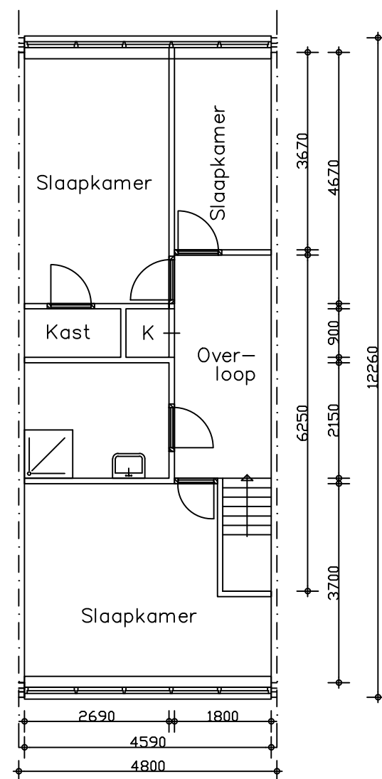
Verdieping
