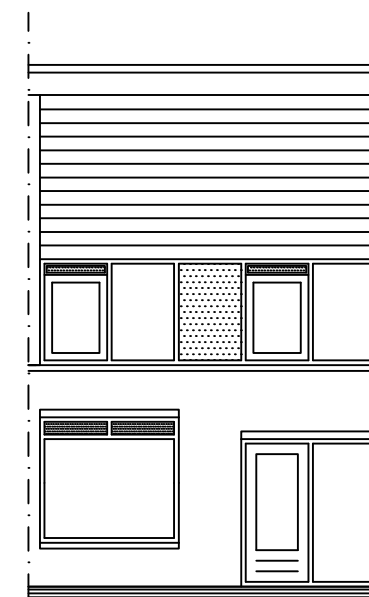
Achtergevel
