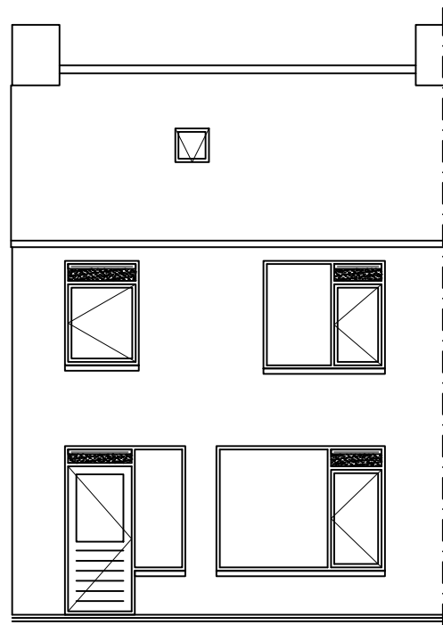
Achtergevel
