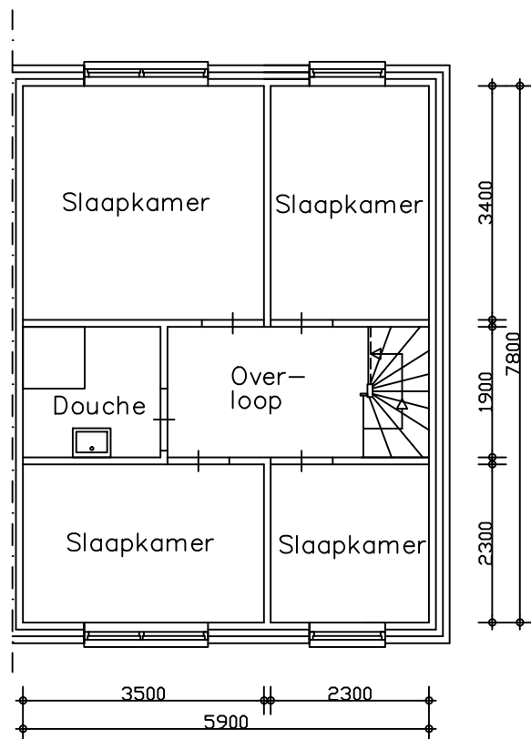
Verdieping
