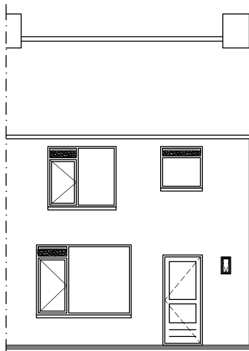
Voorgevel
