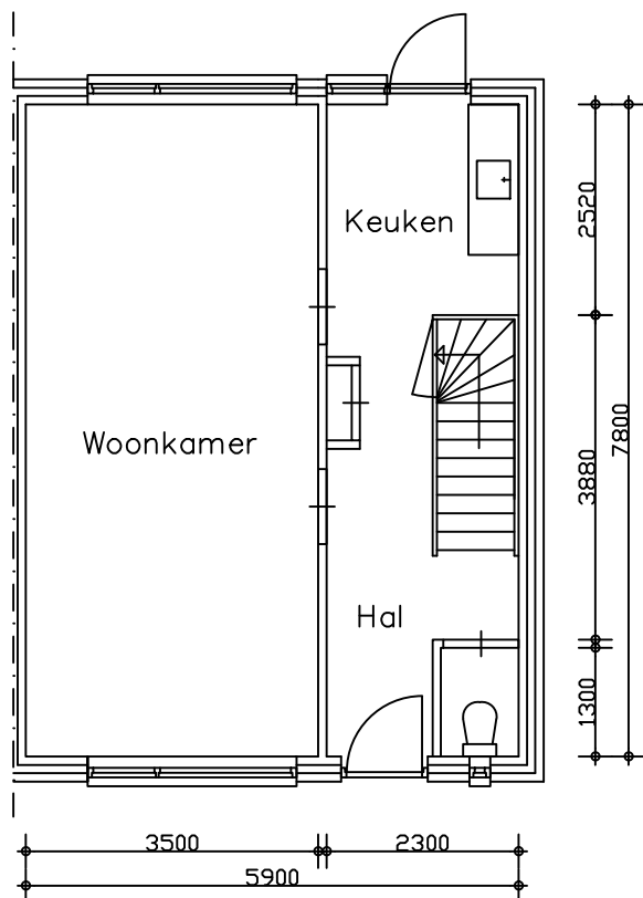
Beganegrond
