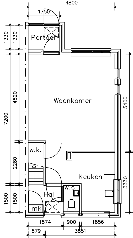
Beganegrond
