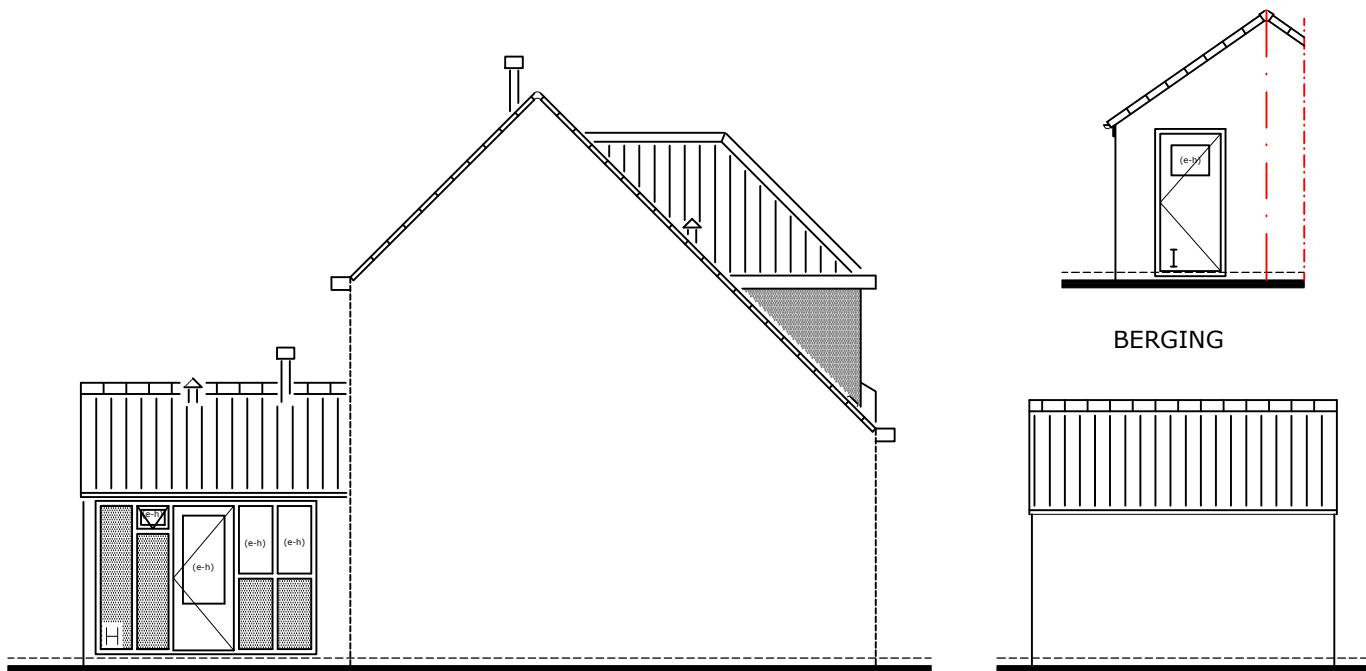
LINKER ZIJGEVEL
