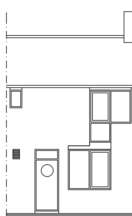
Voorgevel
