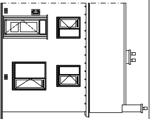
Voorgevel
